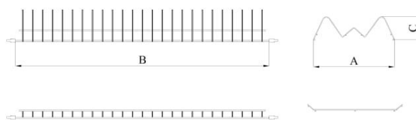
Ociekarka standard
