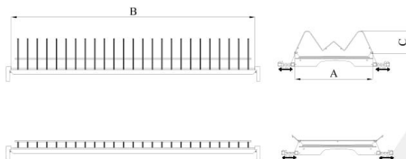
Ociekarka ekonomiczna
